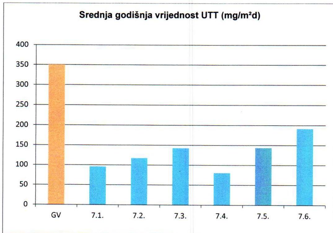
Slika 2. Raspodjela godišnjih vrijednosti UTT za 2024.god. (mg/m 2 d)
